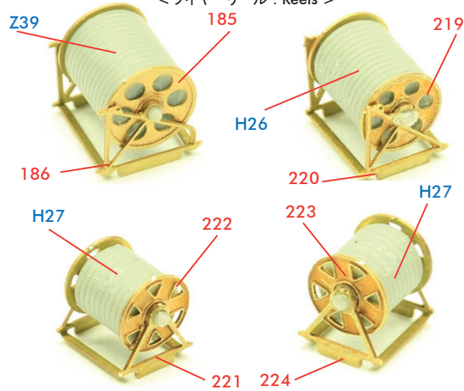
<ワイヤーリール : Reels >
