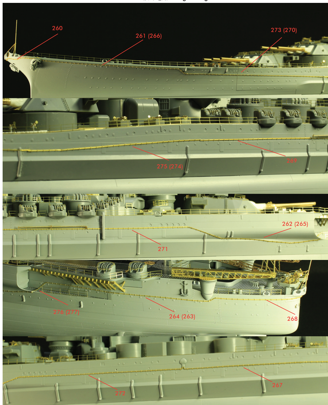
< 舷外電路 : Degaussing Cables >
