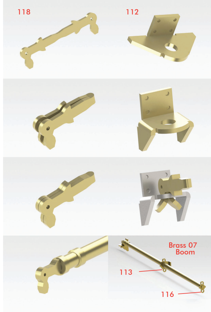
<台車 :Trolley>
