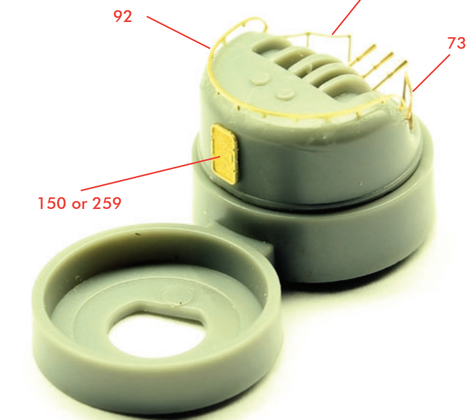
<シールド付き 25mm 3 連装機銃 : 25mm Triple Machine Guns with Shield>
