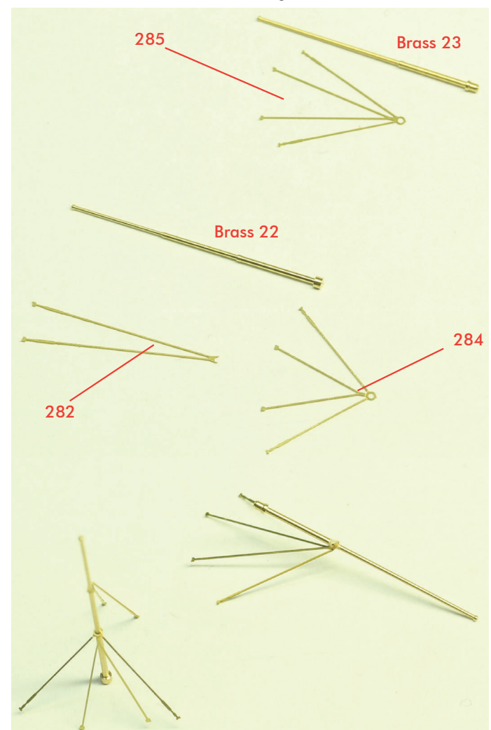
< 船首旗竿/船尾旗竿 : Jack Staff / Ensign Staff >
