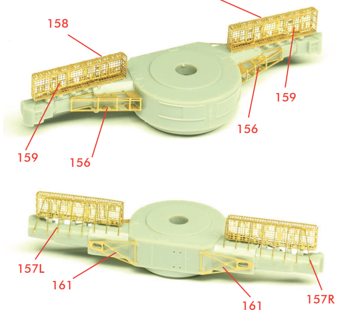
< 二一号電探: 21 Go Radar >
