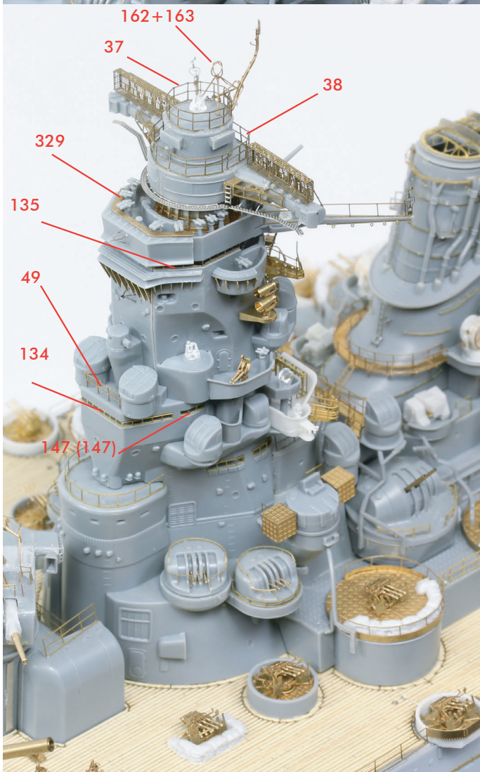
< 信号旗掛: Flag Locker >
