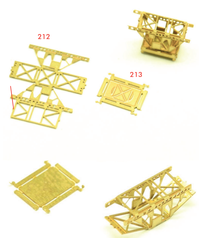
< 台車 : Trolley >
