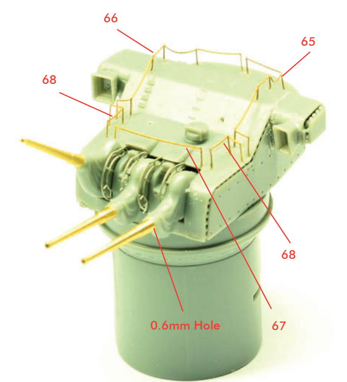
<155mm 三連装 副砲塔 : 155mm Triple Guns>
