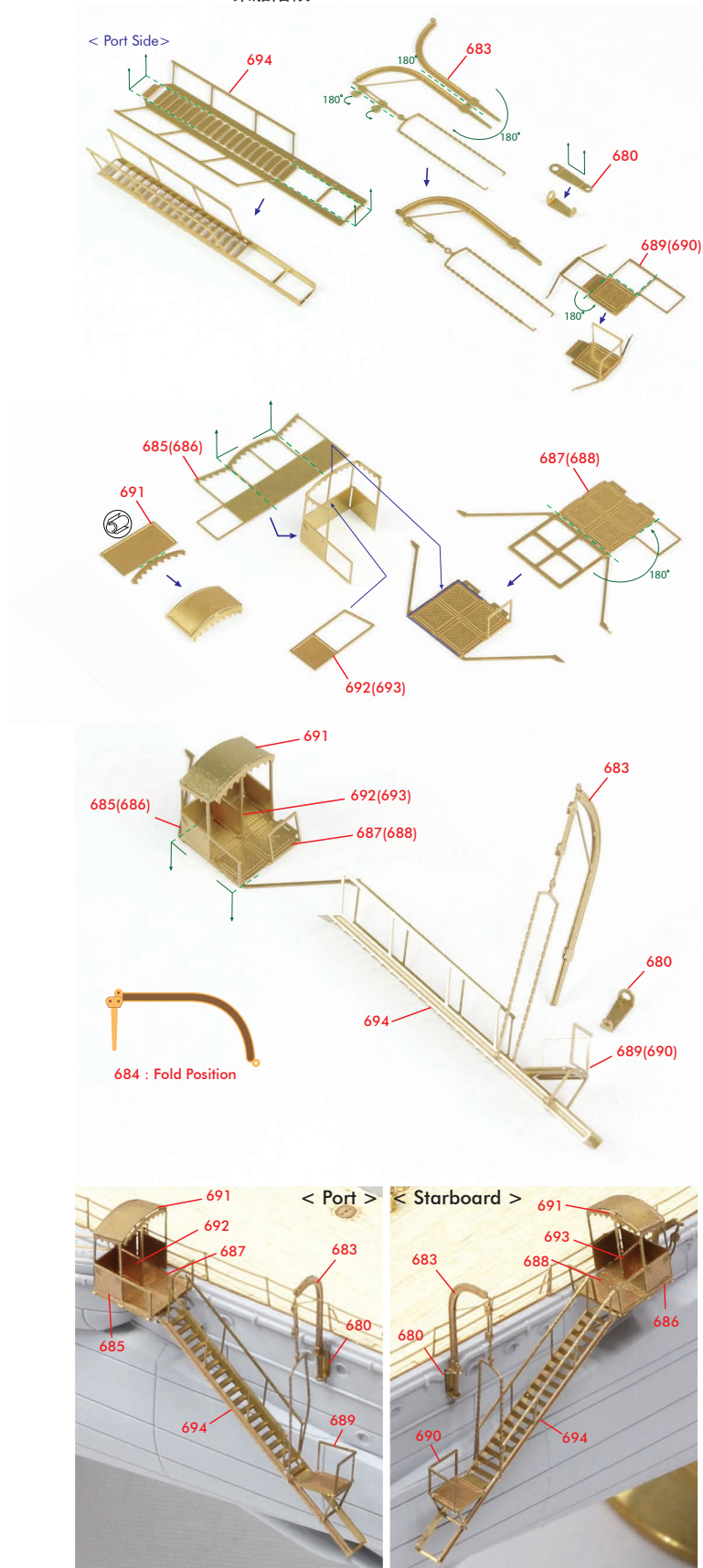
< 乗船階段：Accommodation Ladder >
