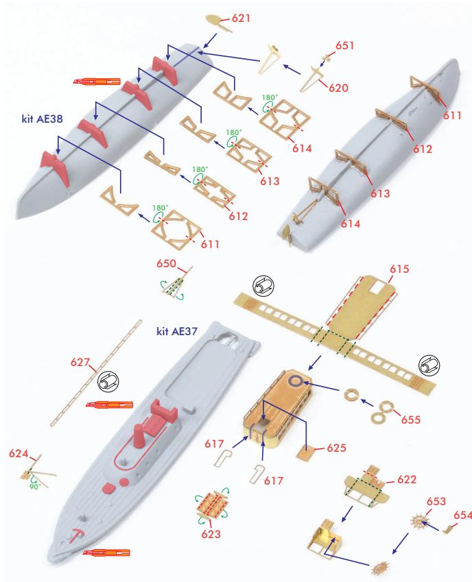
< 17m水雷艇：17m Motor Pinnace >
