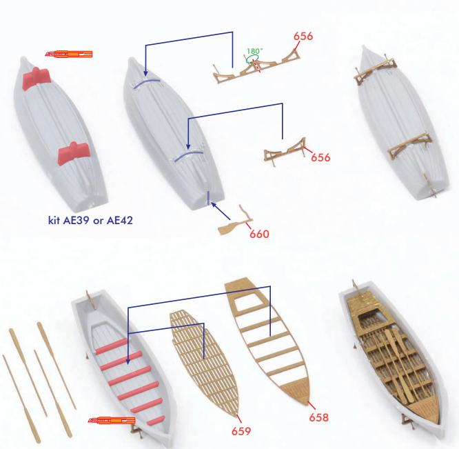
< 9mカッター：9m Cutter >
