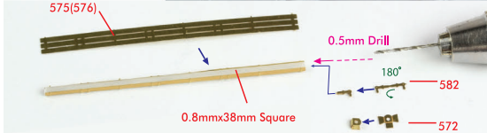
<甲板支柱 : Stanchion 2>
