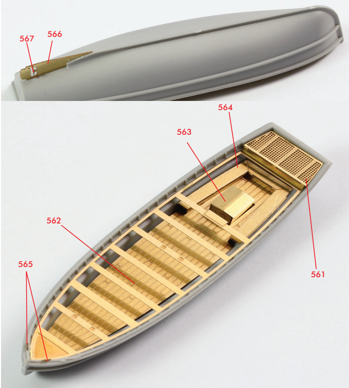
<36ft MOTOR PINNACE>
