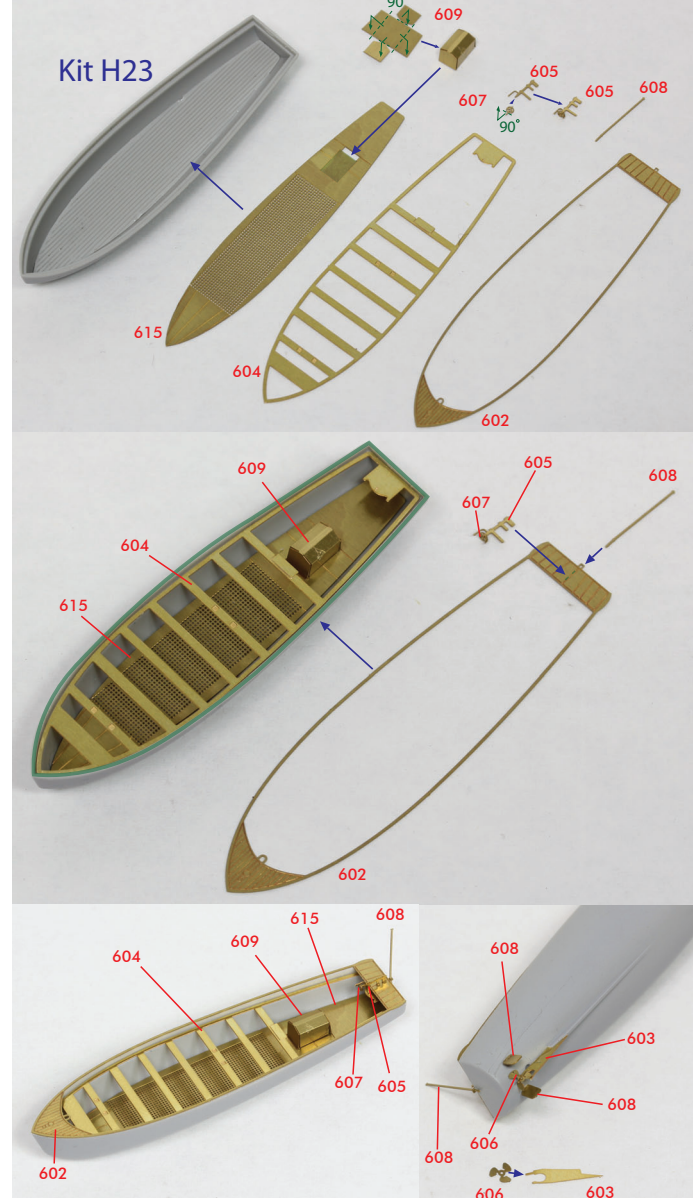
<36ft MOTOR PINNACE>
