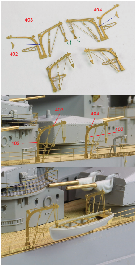
<Davit>
