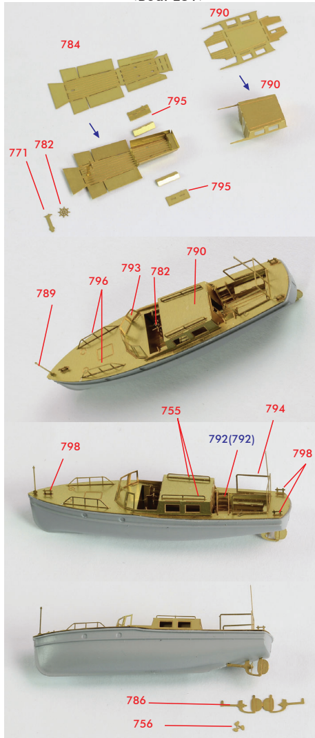
<Boat E31>
