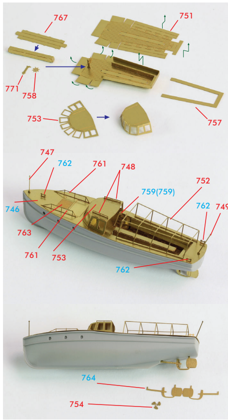
<Boat E31>
