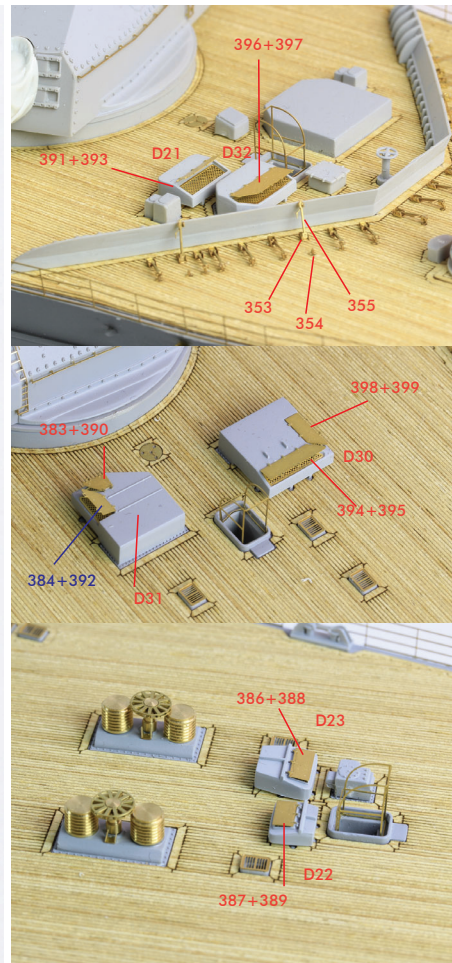
<Ventilator>
